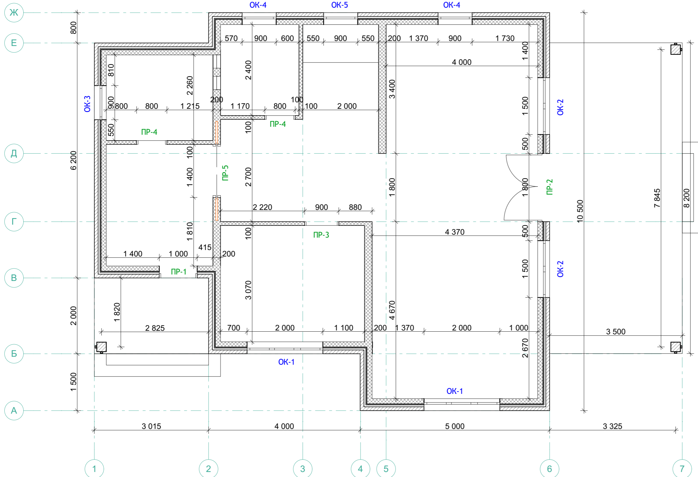
Экспликация проемов первого этажа
